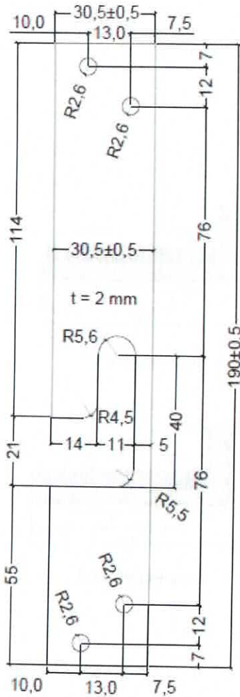
Verstärkungsblech aus Aluminium, t = 2 mm, für Randhöhe 35 mm
