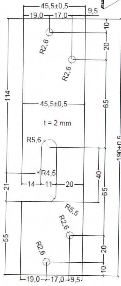
Verstärkungsblech aus Aluminium, t = 2 mm, für Randhöhe 50 mm
